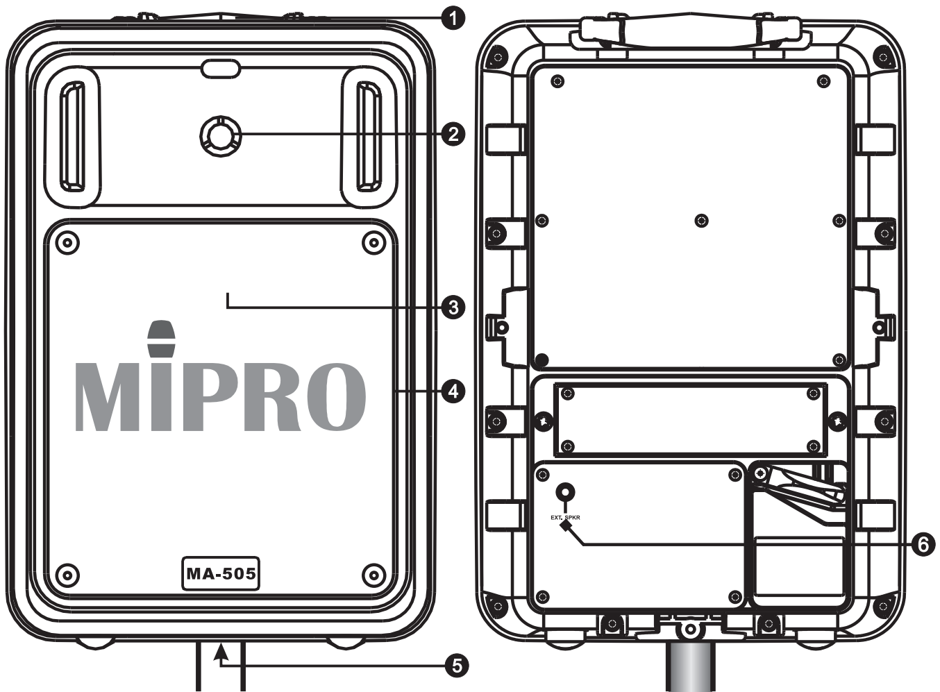
圖 1 : 正面
