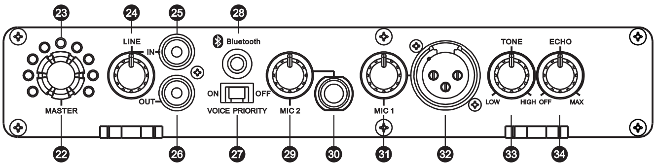
操控面板
