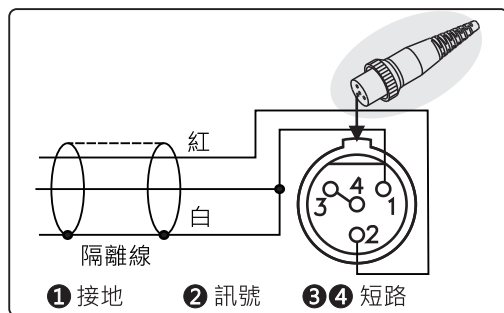
二線式
